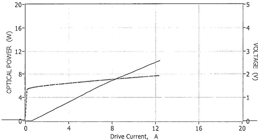
LIV Curve
